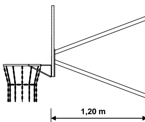
Abb. 2: Basketball-Wandanlage Outdoor, Seitenansicht
