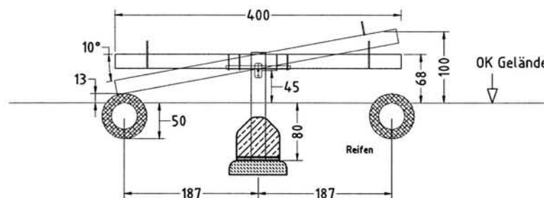
GELÄNDESCHNITT M 1: 50
