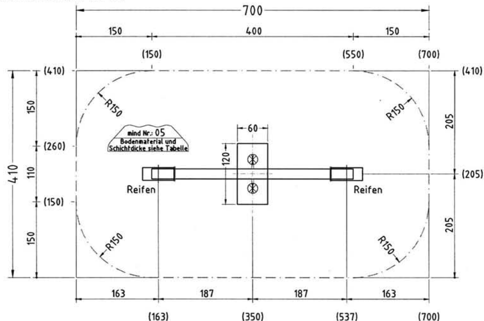
SICHERHEITSBEREICH M 1: 50
