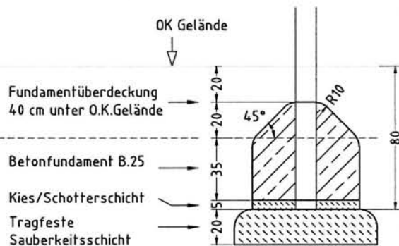
FUNDAMENTSCHNITT M 1: 20
