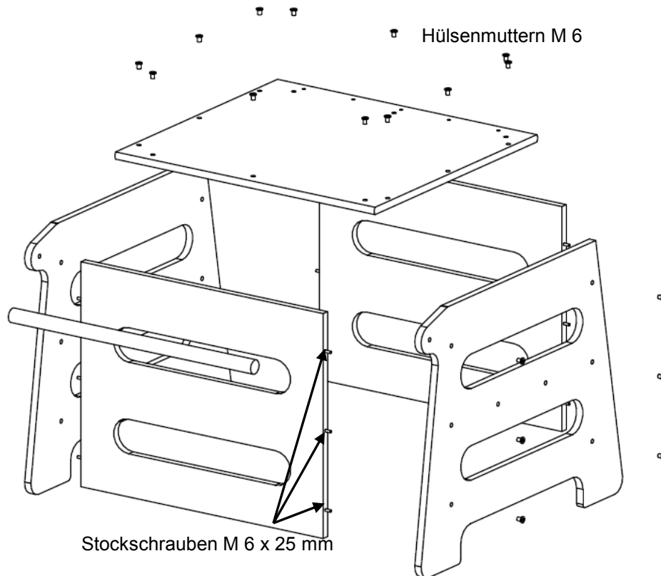
Abb.2 Sport-Thieme Podest - Montagehinweise
