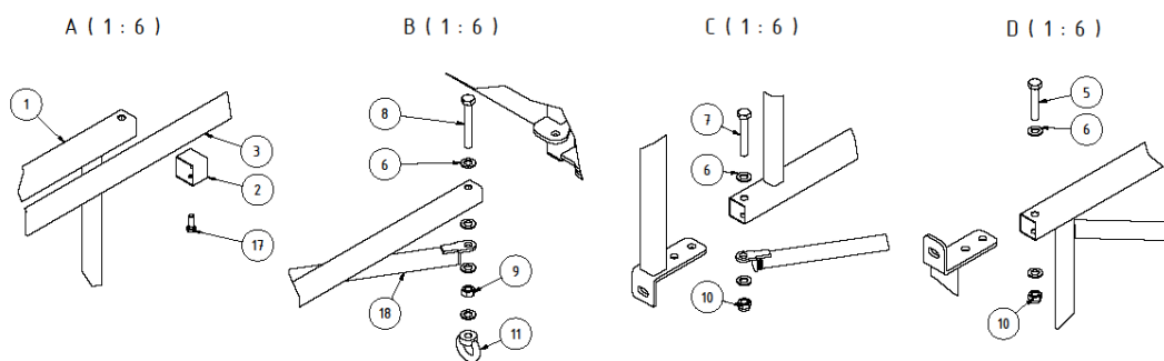
Abbildung 4: Detaillansicht
