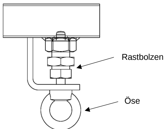
Abbildung 6: Arretierung des Schwenkmechanismus
