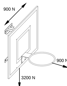
Abbildung 2: Belastbarkeit Basketballbrett
