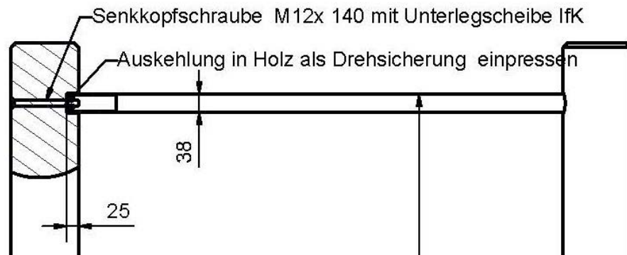
V2A-Stange
