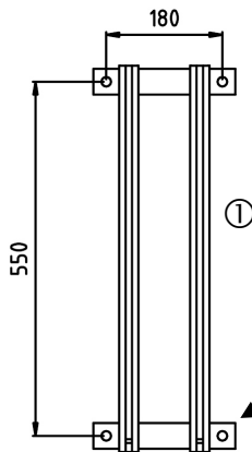
Abb. 2 : Bohrzeichnung
