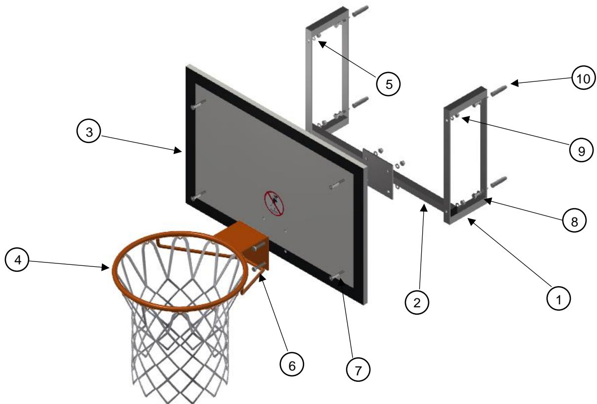
Abbildung 2: Einzelteile der Sport-Thieme Basketball Übungsanlage „starr“
