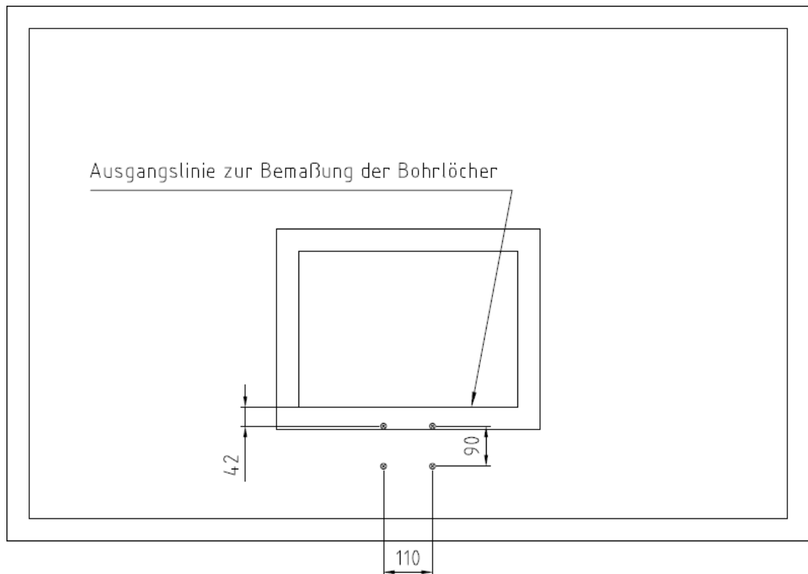
Abb. 5: Bohrmaße
