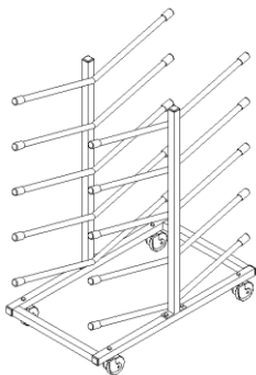
Aufbewahrungswagen (Art.-Nr.: 131 0102)*
