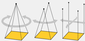
1-Punkt Aufhängung
