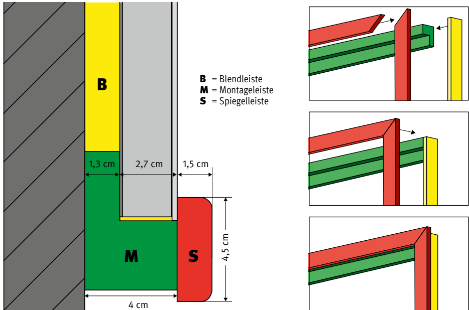
Spiegelleiste
