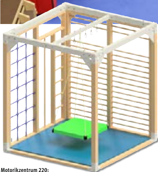
Motorikzentrum 220: 220x220x246 cm, 3 Aufhängeösen.
